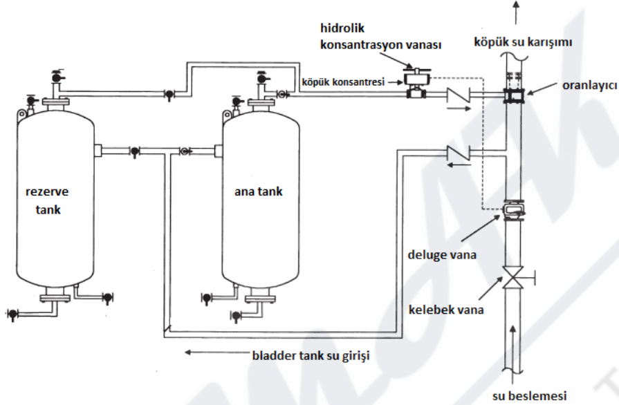
Şekil 2. Yedekli Köpük Tankı Prensip Şeması
